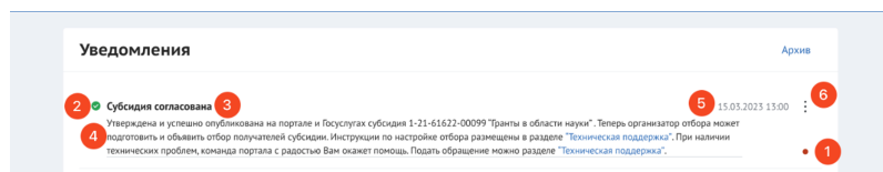
Рисунок 84. Страница «Уведомления»
