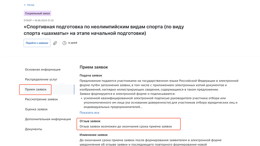
Рисунок 71. Страница отбора
