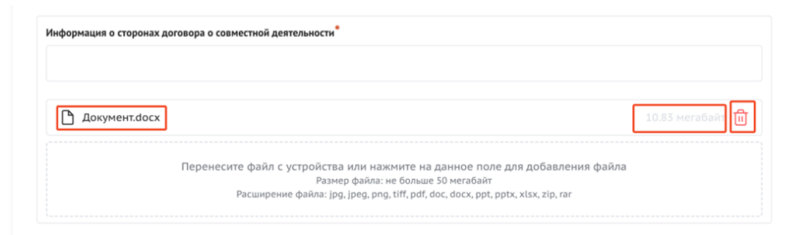
Рисунок 41. Загруженный файл
