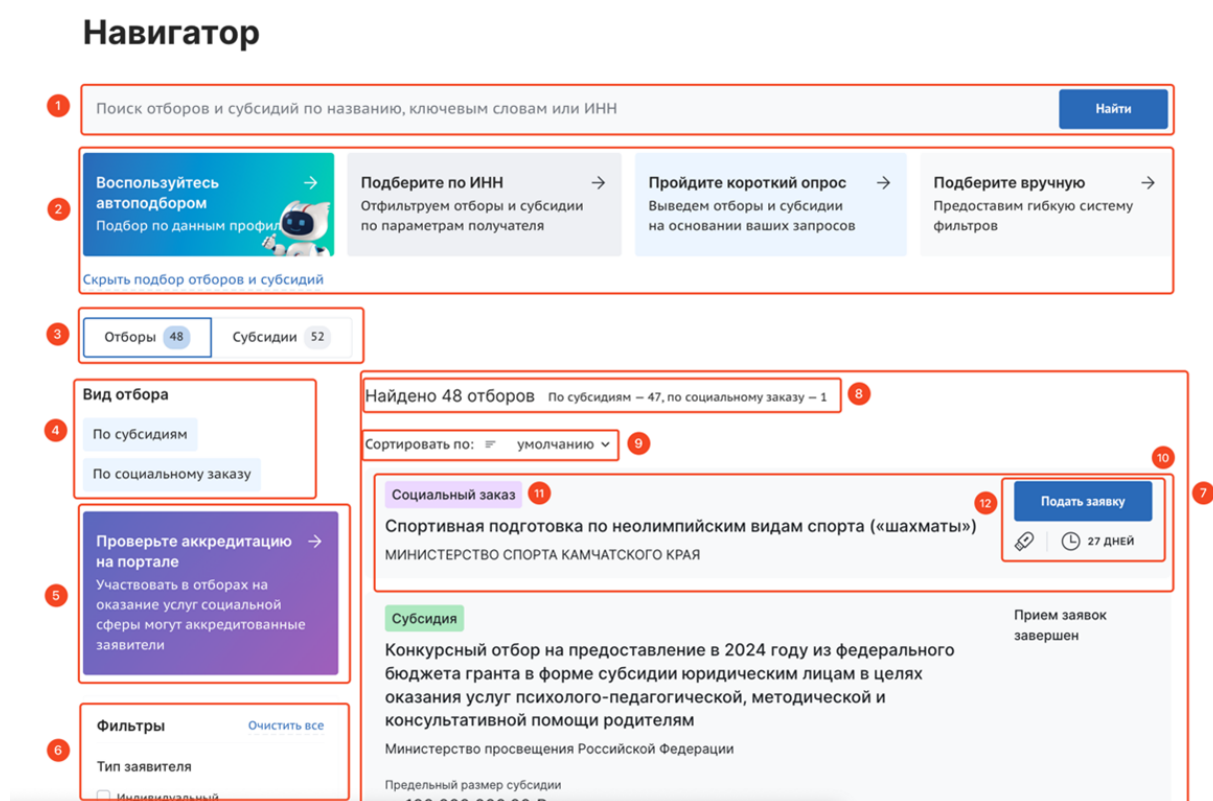
Рисунок 19. «Навигатор»
