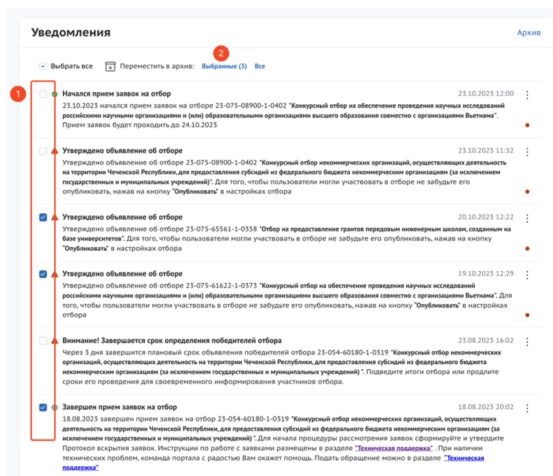
Рисунок 86. Множественный перевод
